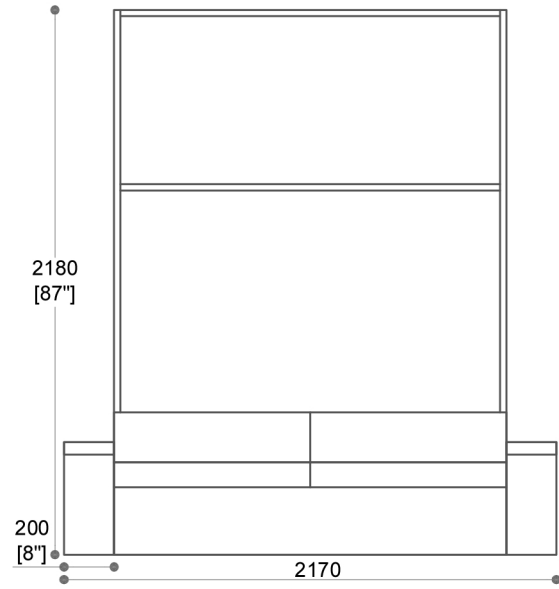
ELEVATION A
